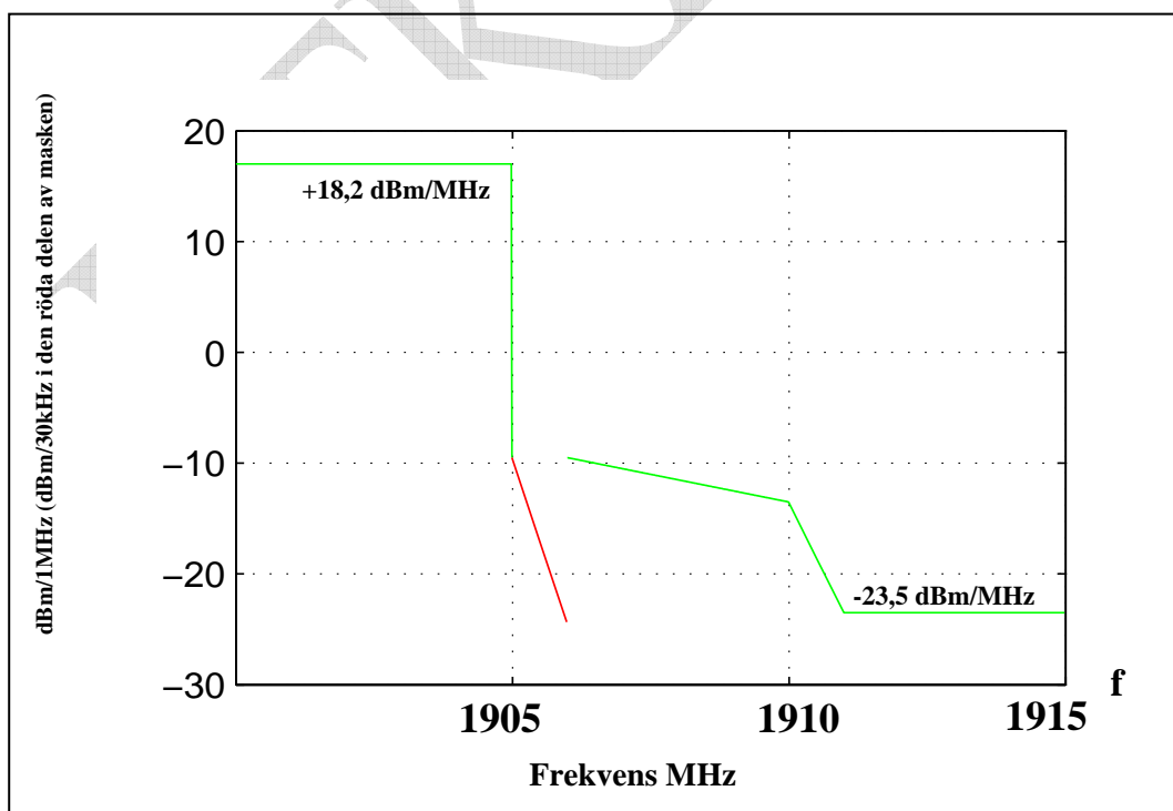
Bild 4: Högsta sändareffekt från terminalen och repeater i upplänksriktning 0 till 10 MHz utanför övre bandkanten.
