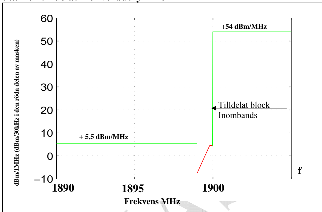
Bild 1: Högsta utstrålade effekt (e.i.r.p.) från basstationssändare och repeater i nedlänksriktning 0 till 10 MHz utanför nedre bandkanten.
