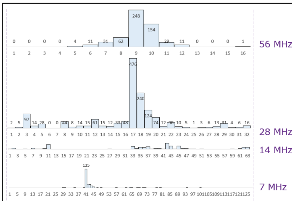
Figur 18), Kanalfördelning i 26 GHz (24500–26500 MHz).
