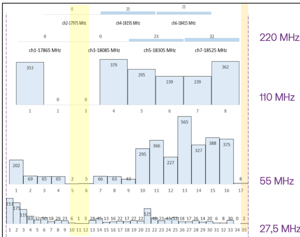
Figur 16) Kanalfördelning i 18 GHz (17700–19700 MHz).
