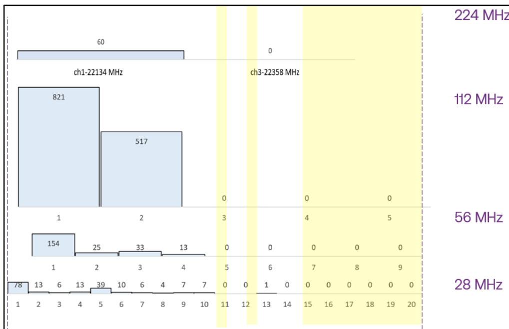
Figur 17) Kanalfördelning i 23 GHz (22000–23600 MHz).
