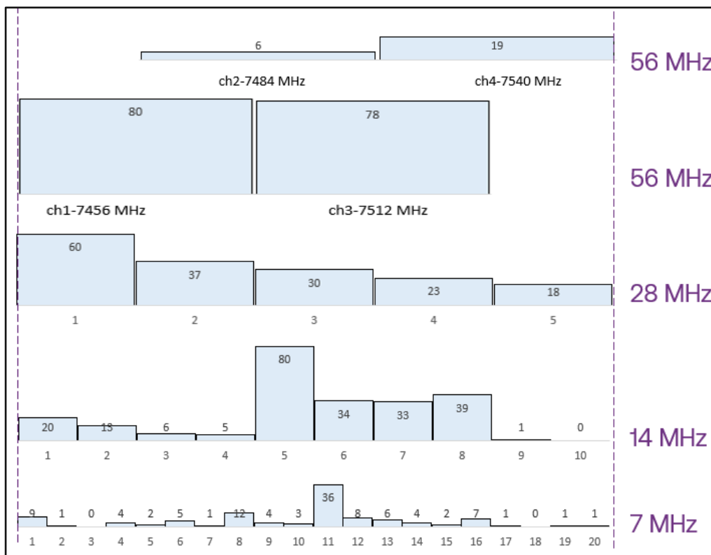
Figur 11) Kanalfördelning i 7 GHz (7425–7725 MHz).
