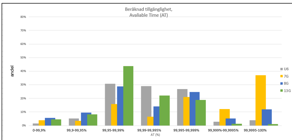
Figur 29, Procentuell fördelning 6–13 GHz.
