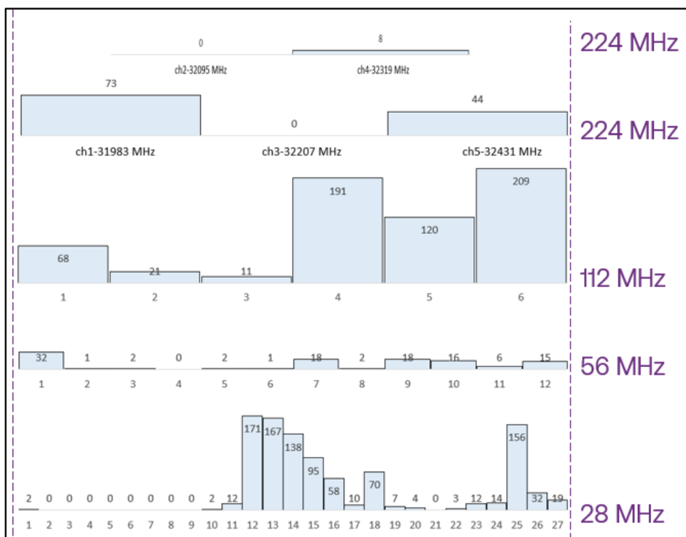
Figur 19) Kanalfördelning i 32 GHz (31800–33400 MHz).
