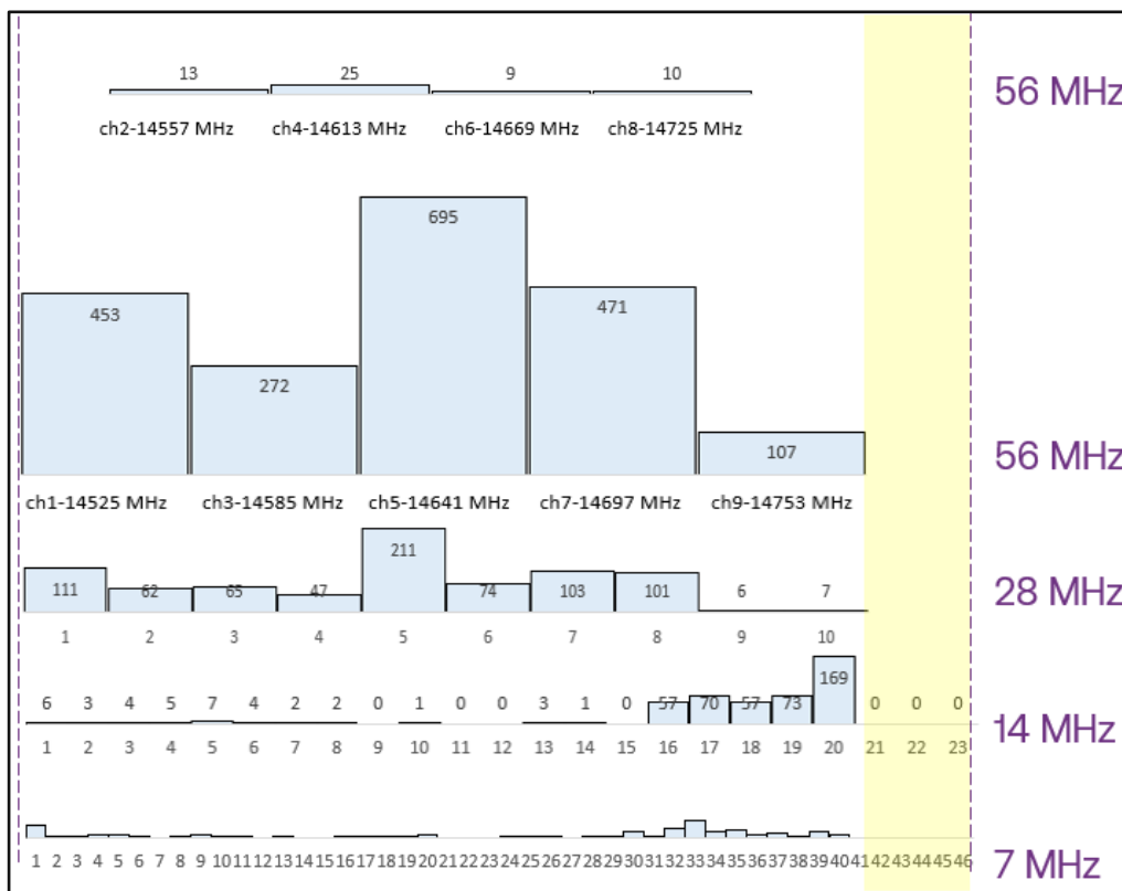
Figur 15) Kanalfördelning i 15 GHz (14500–15250 MHz).
