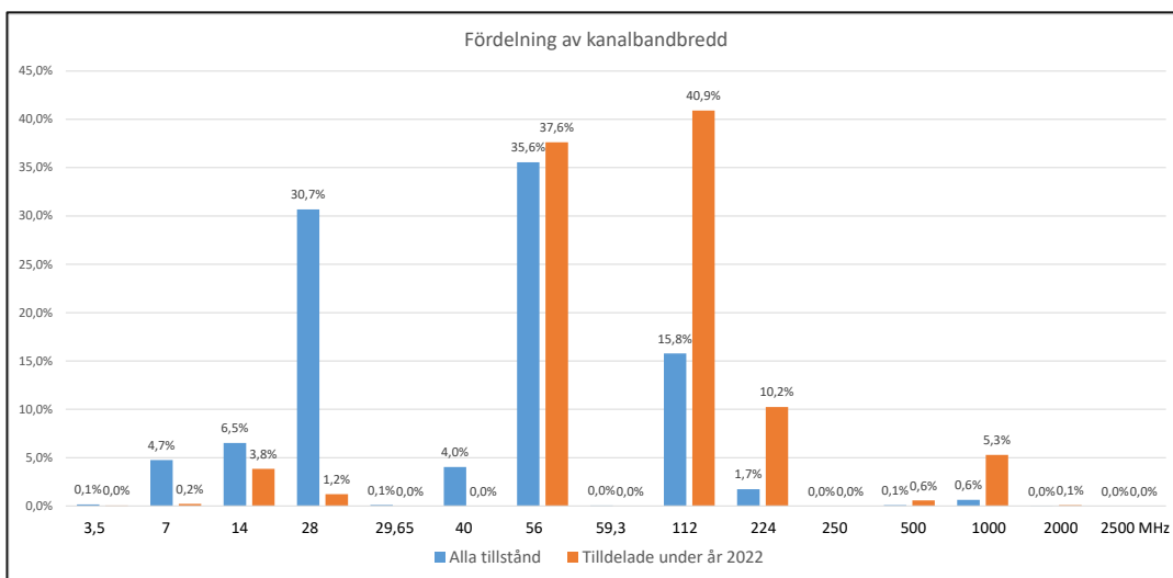
Figur 10) Jämförelse av procentuell andel av kanalbandbredd för alla länkar (ljusblå stapel) och nyansökningar för 2022 (orange stapel).
