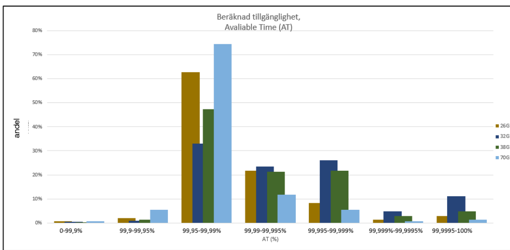
Figur 31, Procentuell fördelning 26–70/80 GHz.
