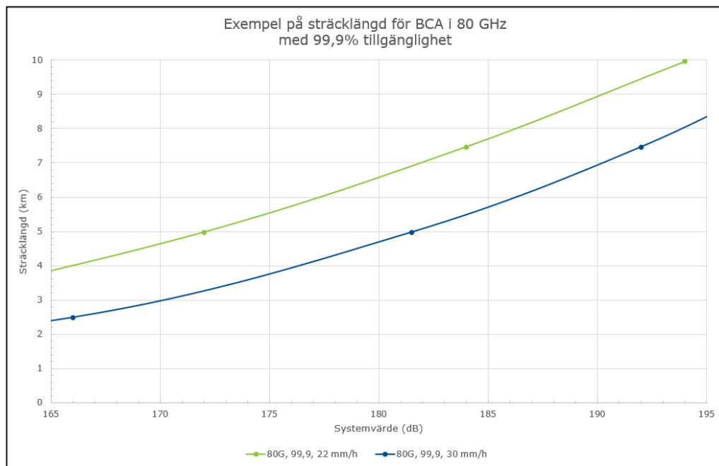
Figur 33. Sträcklängd som funktion av systemvärde vid regnintensitet A0.01 = 22 mm/h respektive 30 mm/h med vertikal polarisation, tillgänglighetskrav 99,9% för BER 10 -6 .
