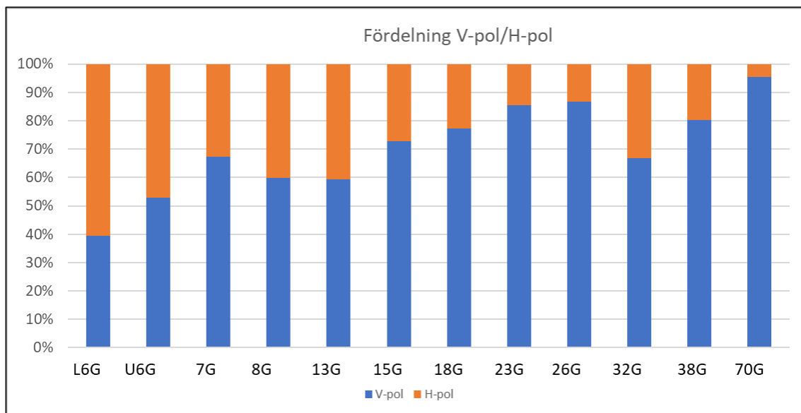
Figur 3) Fördelning av polarisation (V-blå, H-röd) år 2021. Vid framtagande av ovanstående bild fanns inga enskilda tillstånd i frekvensbanden 10,5 GHz eller 28 GHz.
