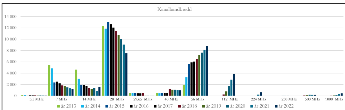
Figur 9) Tilldelad kanalbandbredd fördelat per år.
