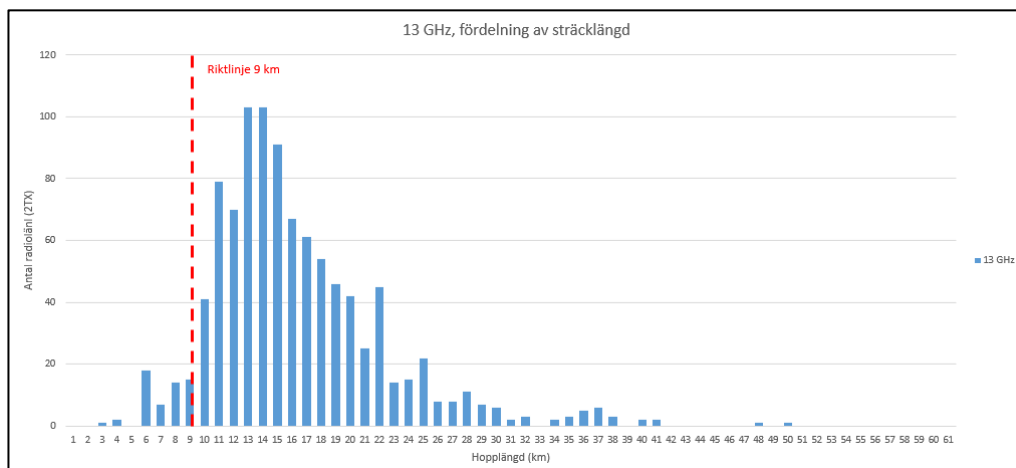
Figur 24) Fördelning av sträcklängd i 13 GHz.
