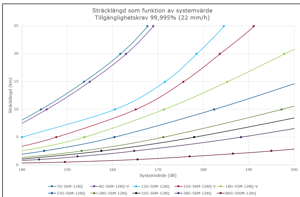
Figur 4) Sträcklängd som funktion av och systemvärde vid regnintensitet A_{0,01} = 22 mm/h med vertikal polarisation, tillgänglighetskrav 99,995% för BER 10 -6 .
