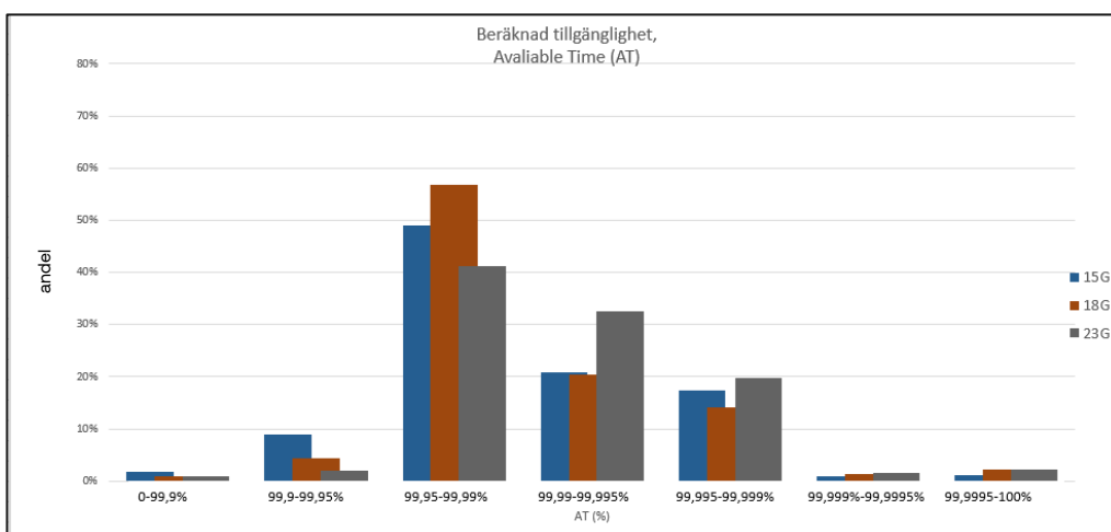
Figur 30, Procentuell fördelning 15–23 GHz.
