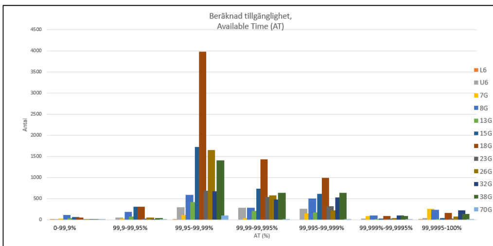
Figur 28, Beräknad tillgänglighet 6–80 GHz (antal fast radio, 2TX/fast radio).
