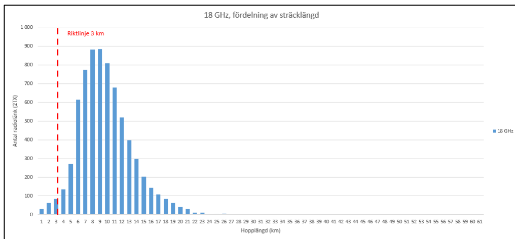
Figur 26) Fördelning av sträcklängd i 18 GHz.
