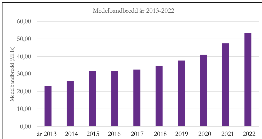
Figur 7) Medelbandbredd för fast radio (fast radio) mellan 6–38 GHz i Sverige. Frekvensbandet 70/80 MHz ingår inte vid beräkning av medelbandbredd eftersom de mycket breda kanalbandbredderna 250/500/1000/2000 MHz annars får en kraftig inverkan på resultatet.
