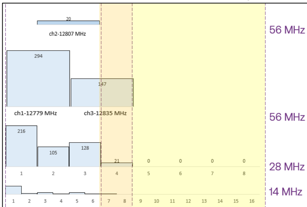
Figur 14) Kanalfördelning i 13 GHz (12750–13250 MHz).
