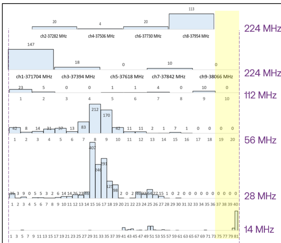
Figur 20) Kanalfördelning i 38 GHz (37000–39500 MHz).
