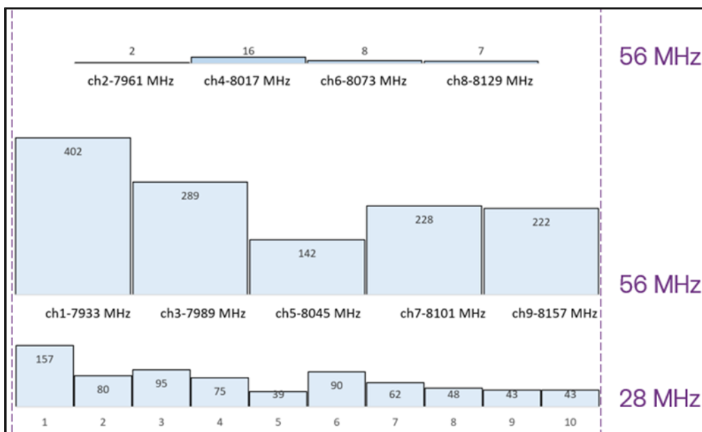
Figur 12) Kanalfördelning i 8 GHz (7900–8500 MHz).
