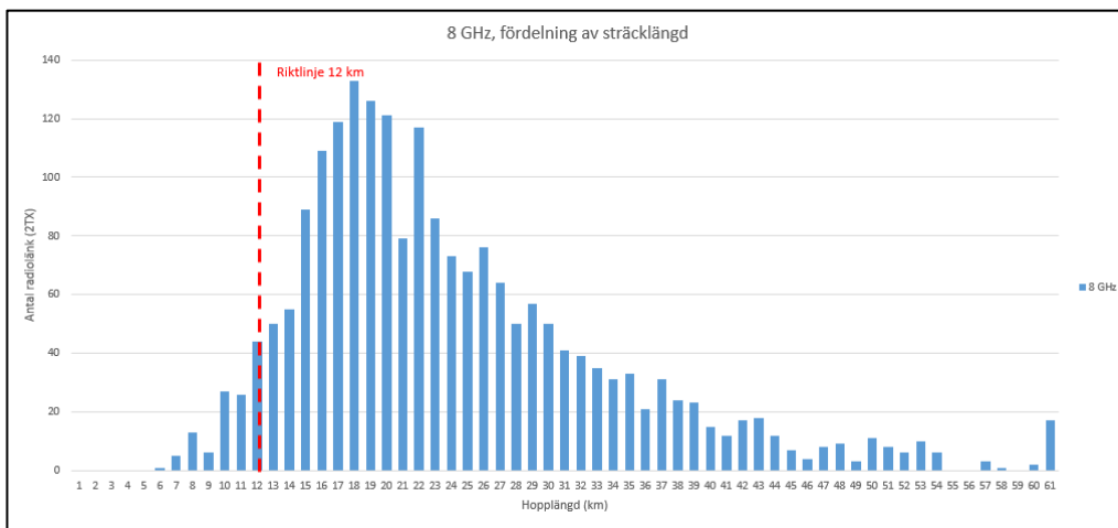
Figur 23) Fördelning av sträcklängd i 8 GHz.
