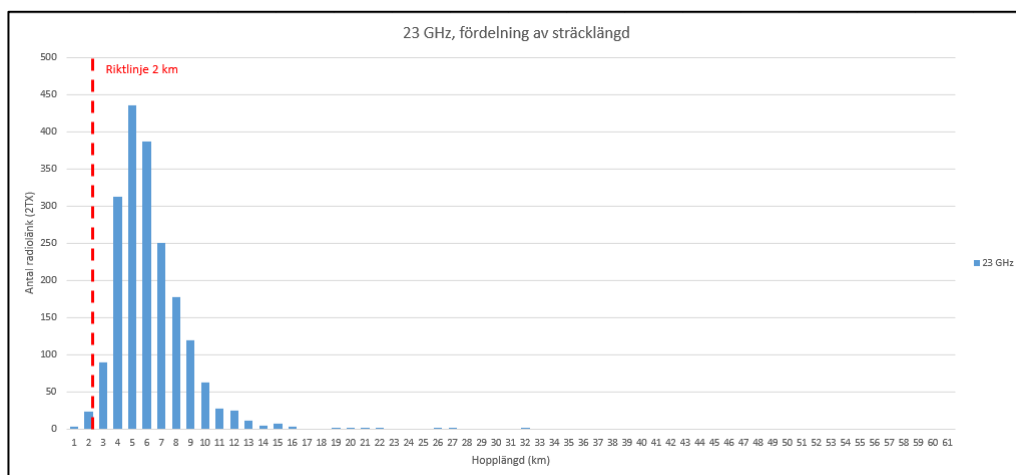
Figur 27) Fördelning av sträcklängd i 23 GHz.
