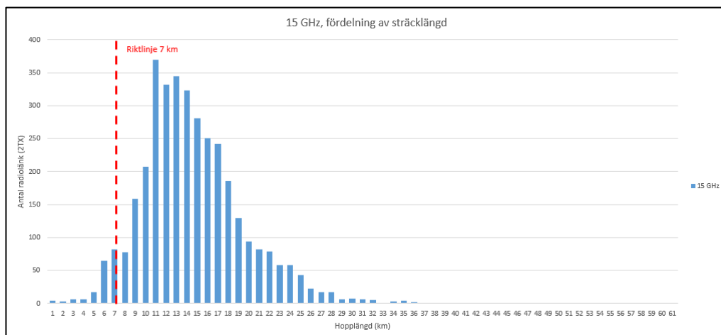
Figur 25) Fördelning av sträcklängd i 15 GHz.
