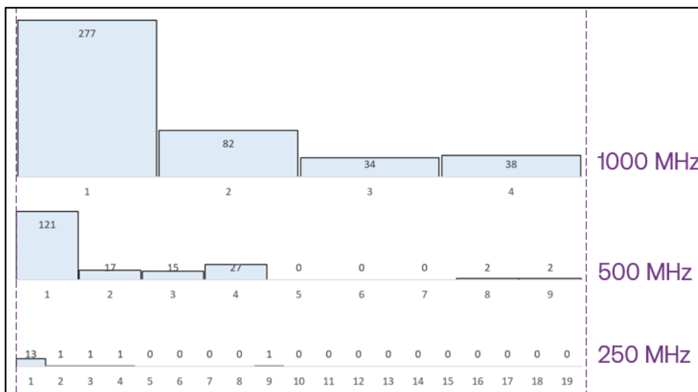
Figur 21) Kanalfördelning i 70/80 GHz (71000–86000 MHz).
