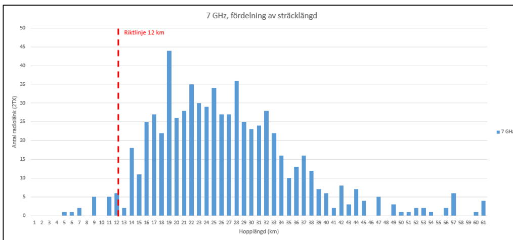
Figur 22) Fördelning av sträcklängd i 7 GHz.
