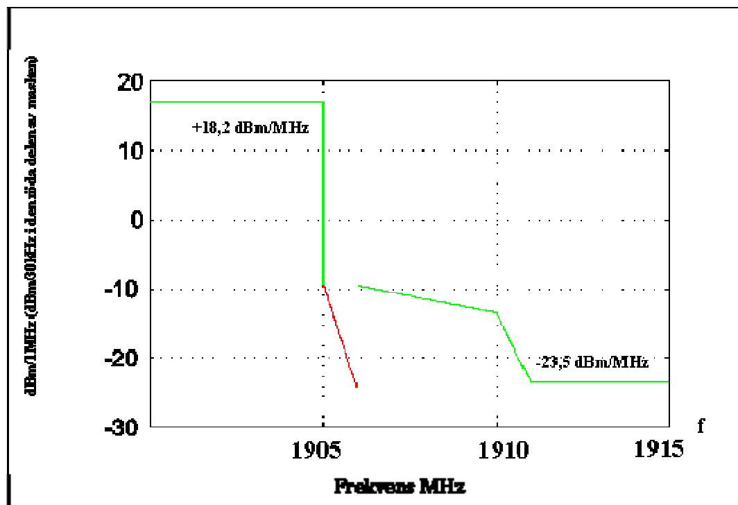
Bild 4: Högsta sändareffekt från terminalen och repeater i upplänksriktning 0 till 10 MHz utanför övre bandkanten.
